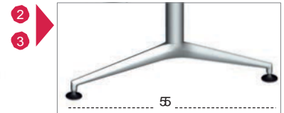
columna cilíndrica de acero Ø60 x 2 mm pie de aluminio inyectado de 55 cm x 6 mm
